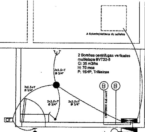
INSTALACIÓN ELÉCTRICA
