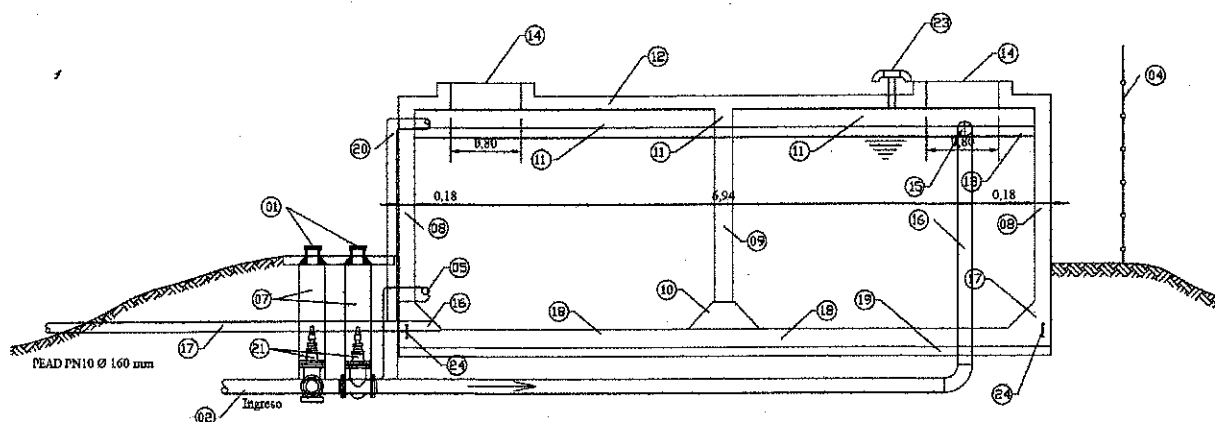
CORTE TRANSVERSAL A-A
